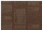
7358 Breccia
